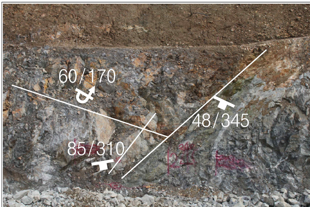
【그림 23】 B 영역에 발달한 불연속면
